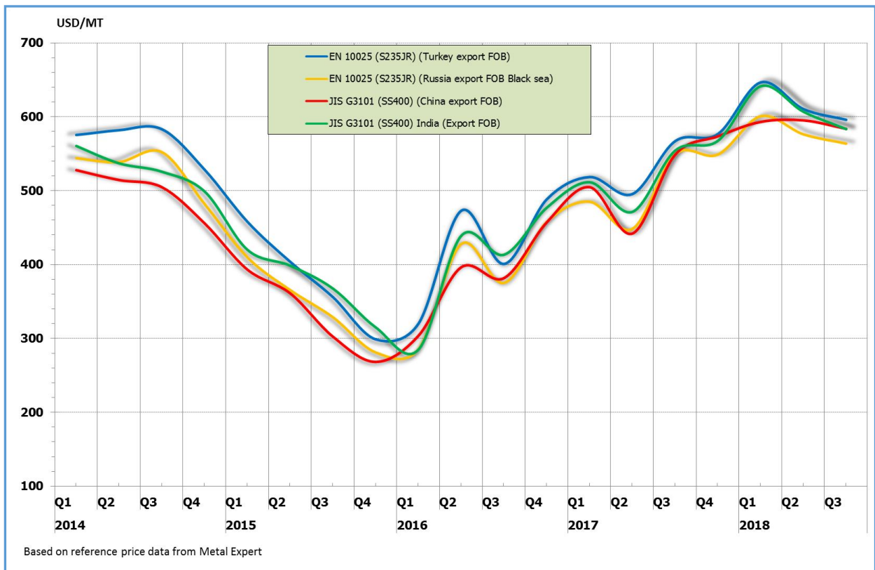
กราฟแสดงราคาเหล็กแผ่นรีดร้อนชนิดม้วนอ้างอิงในตลาดโลก ช่วงไตรมาส 1/2557 - ไตรมาส 3/2561
