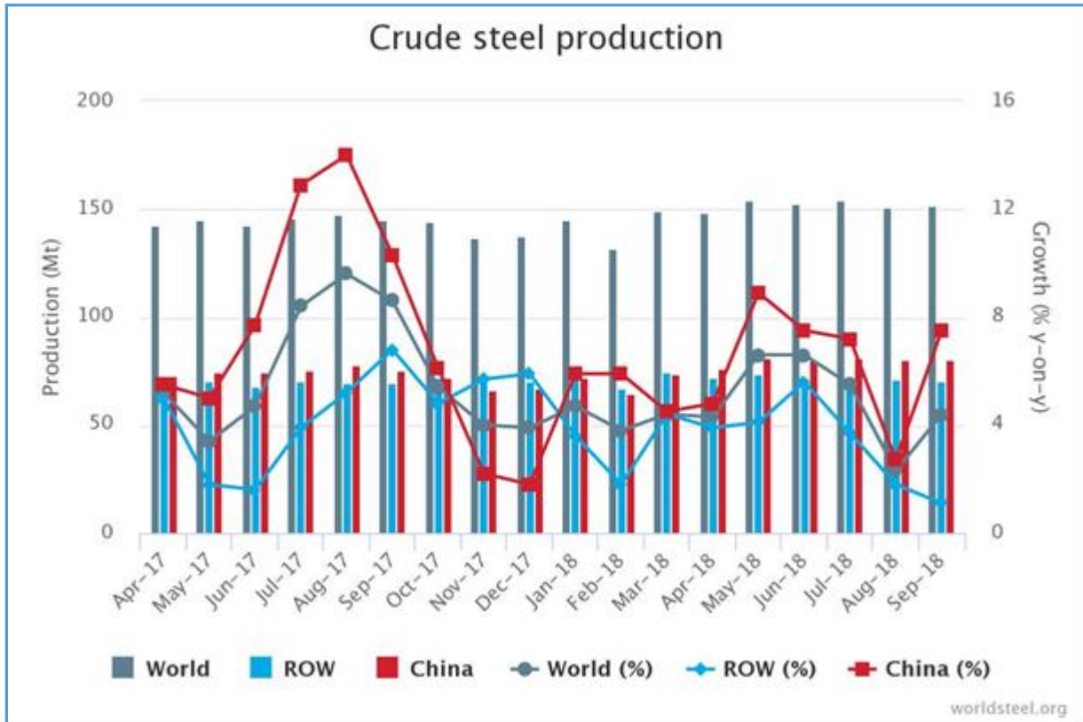
กราฟแสดงปริมาณการผลิตเหล็กดิบของโลก สิ้นสุด ณ 30 กันยายน 2561
