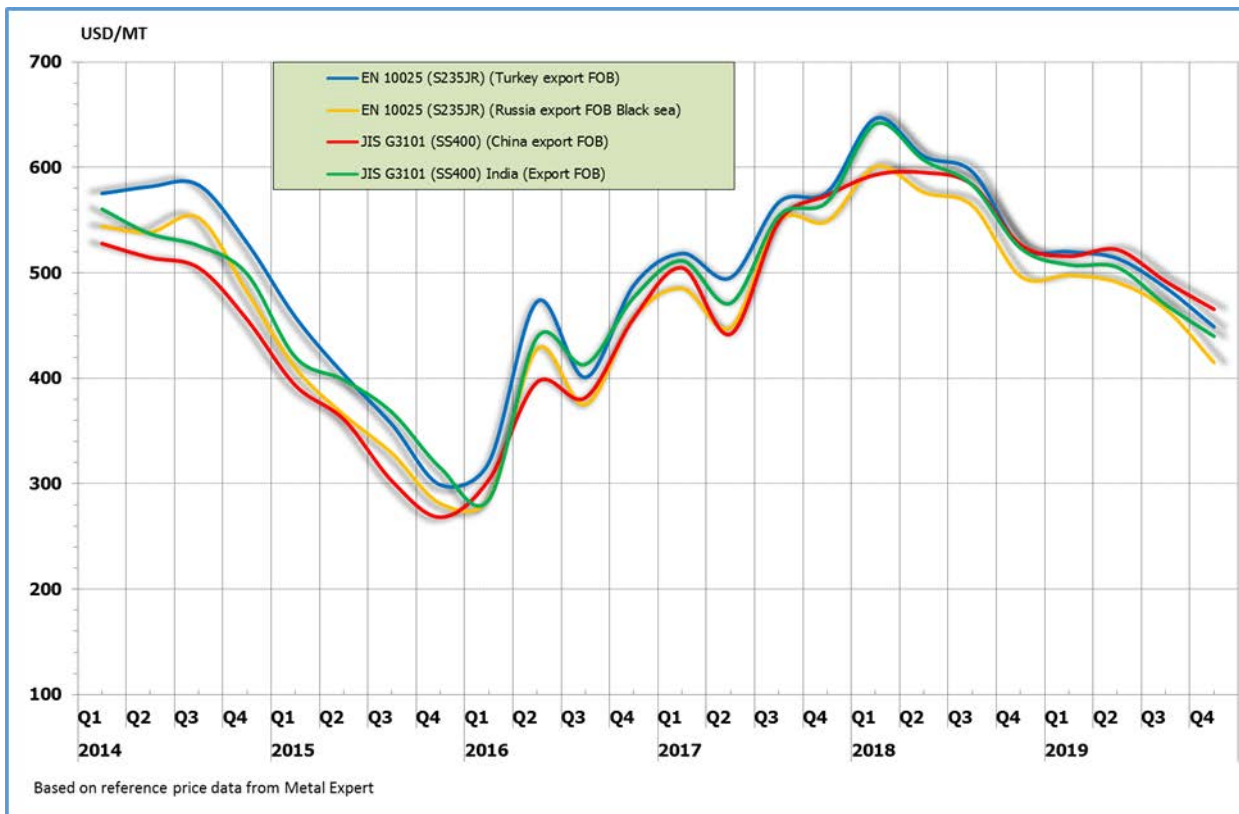
กราฟแสดงราคาเหล็กแผ่นรีดร้อนชนิดม้วนอ้างอิงในตลาดโลก ช่วงไตรมาส 1/2557 - ไตรมาส 4/2562
