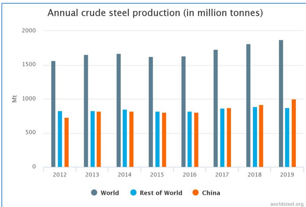
กราฟแสดงปริมาณการผลิตเหล็กดิบของโลก สิ้นสุด ณ 31 ธันวาคม 2562
