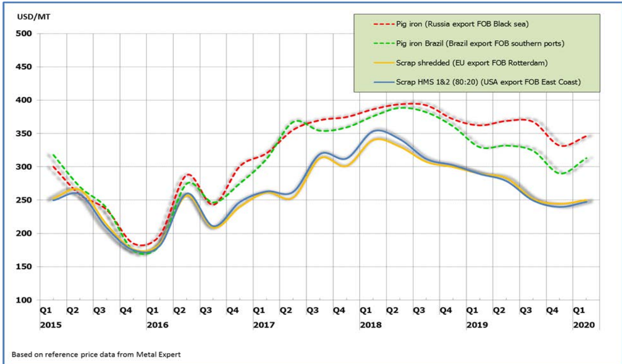
กราฟแสดงราคาวัตถุดิบอ้างอิงในตลาดโลก ช่วงไตรมาส 1/2558 - ไตรมาส 1/2563
